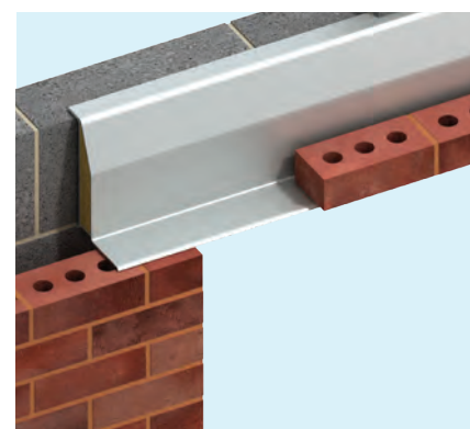
Ancon Lintel
