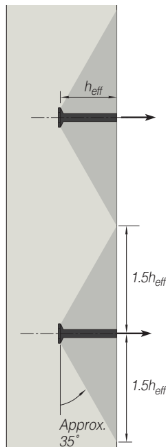
Fig A. Full Tensile Cone
